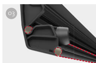
Versteckte Kederschienen zur Anbringung des Vorzelt Room Van Premium oder anderes Zubehör
