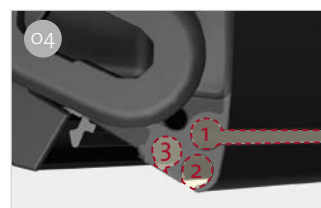
Driedubbele geleider Voor montage van een frontpaneel of de Privacy en andere accessoires
